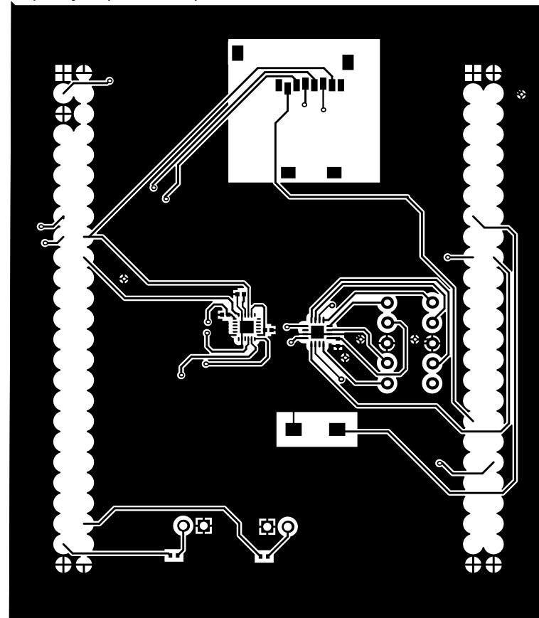
Top Layer (Scale 3:2)
